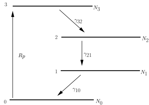
Figure 1: Energieniveaudiagramm für Nd:YAG Die beim Übergang 2 \rightarrow 1 ausgesendeten Photonen gelangen in den Resonator der eine Reflexionsrate von T_R = 99\% aufweist. Die Intensität der Strahlung im Medium ist durch I = cnh\nu_0/V_{\text{Laser}} gegeben ( c Lichtgeschwindigkeit, n Anzahl Photonen im Resonator, V_{\text{Laser}} = 5\text{mm}^3 Volumen des Lasers). Daraus ergibt sich die Wahrscheinlichkeit für die stimulierte Emission zu W_{\text{stim}} = \sigma I/h\nu_0 , wobei der Wirkungsquerschnitt \sigma für die stimulierte Emission 2 \rightarrow 1 durch \sigma = 6,5 \cdot 10^{-19}\text{cm}^2 gegeben ist. Stelle Ratengleichungen für das Vier-Niveausystem auf, d.h. Differentialgleichungen für die Besetzungszahlen N_i . Zum Beispiel gilt für N_2 : dN_2/dt =
