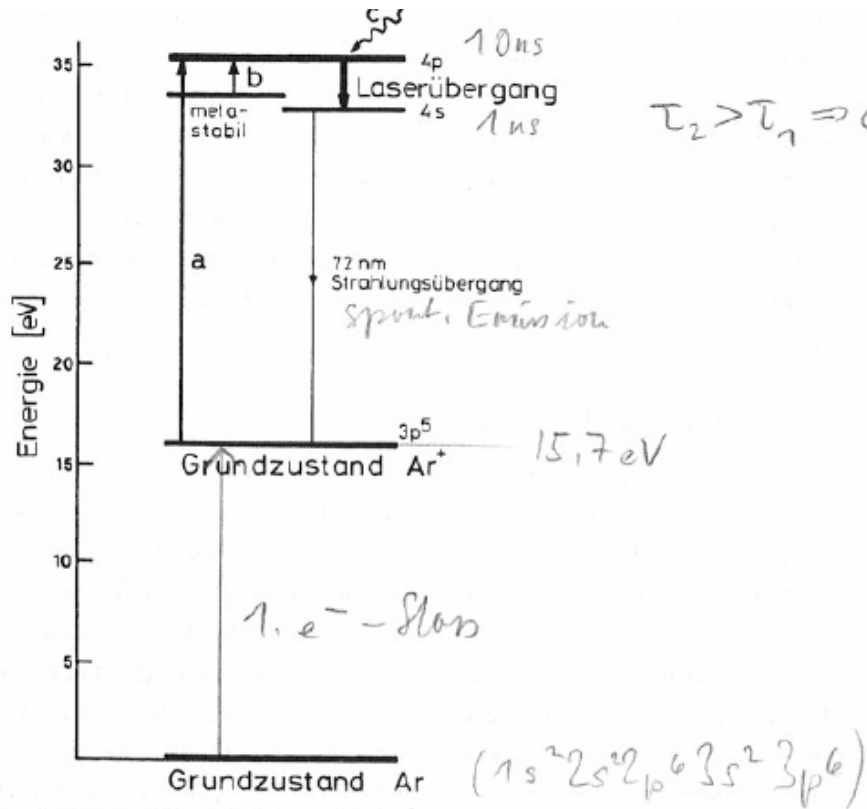
12-6 Energieniveauschema von \text{Ar}^+
