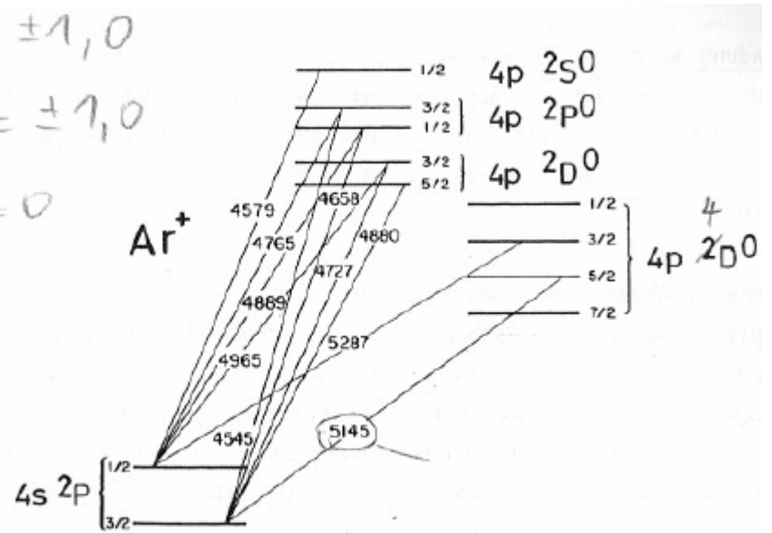
Fig. 12-7 \text{Ar}^+ -Laserübergänge mit Wellenlängen in Å [nach Bridges 1982]
